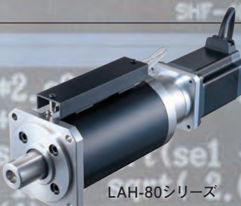
リニアアクチュエーター
